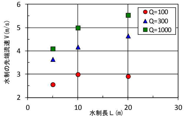
図-3 水制長と先端流速 [Case1, 流速値は絶対値]
