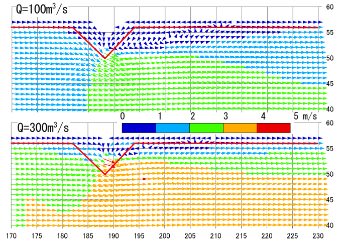
図-2 流速ベクトル図 [Case1]
