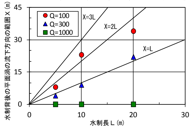
図-4 水制長と渦の範囲 [Case1]
